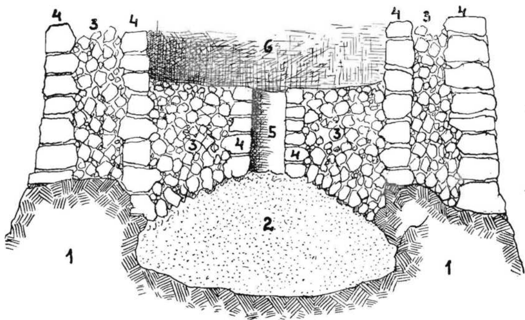
Sl. 12. Grad Borač: vertikalni presjek temelja kule s cisternom (šematični prikaz); 1 prirodna stena, 2 piesak, odnosno šupljina cisterne, 3 kaša lomljenog kamena i maltera, 4 oplata zidova, 5 rupa kroz koju se uzimala voda, 6 podrumski prostor nad cisternom.
